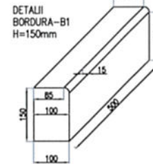
DETALII BORDURA B1 - 10x15
