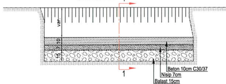
Sectiunea 2-2
