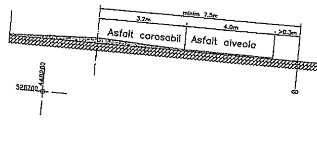
Seiune 1 Scara 1:100
