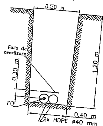
Profil Sant Scara 1:20
