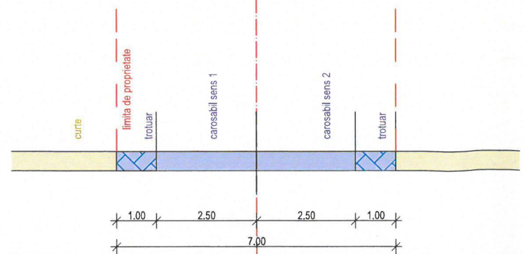
sectiune transversala drum de exploatare propus spre supralargire pana la latimea de 7.00m
